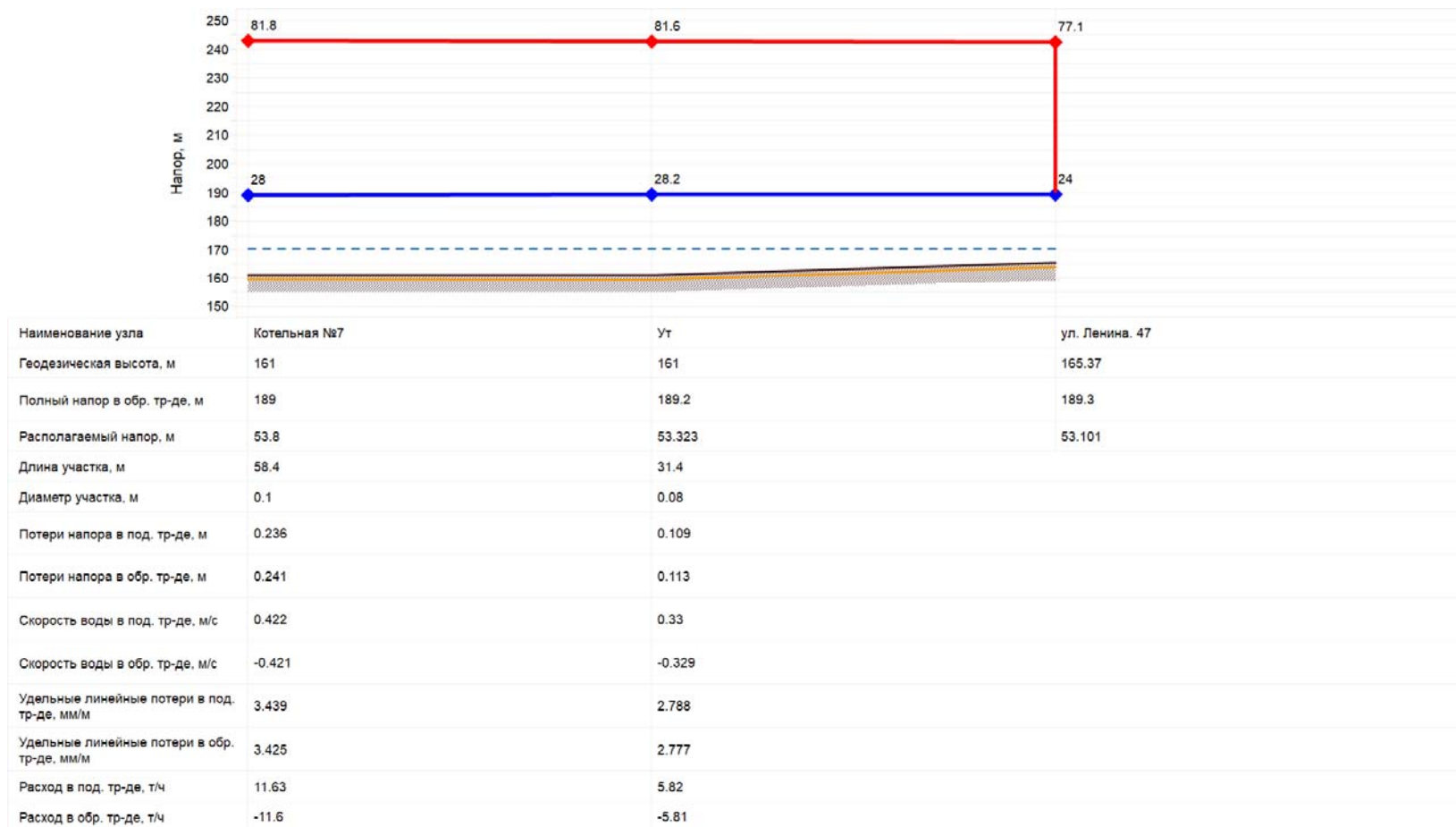
Рисунок 1.18 – Пьезометрический график для участка тепловых сетей от котельной №7 – ул. Ленина, 47
