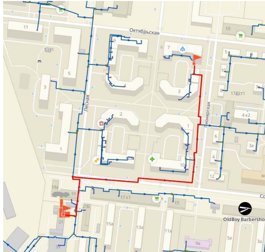
Рисунок 1.15 – Путь пьезометрического графика для участка тепловых сетей от котельной №14 – ИТП Жилой дом (ул. Октябрьская, 7)
