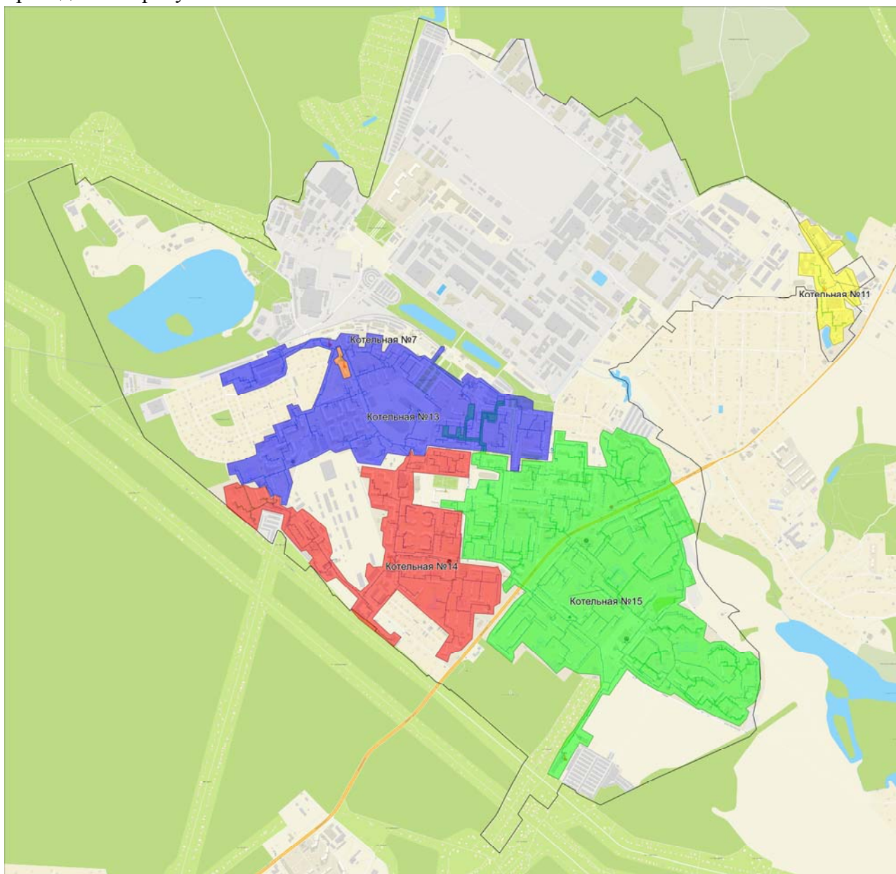
Рисунок 1.3 – Зоны действия источников теплоснабжения, эксплуатируемых на территории г.о. Фрязино
