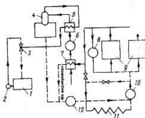
Тепловая схема водогрейной котельной с закрытой системой горячего водоснабжения. 1 — бак расходной воды; 2 — эжекторный насос; 3 — эжектор; 4 — вакуумный деаэрактор; 5 — охладитель пара; 6 — химводоочистка; 7 — теплообменник; 8 — рециркуляционный насос; 9 — котел; 10 — циркуляционный сетевой насос; 11 — теплосеть; 12 — подпиточный насос
