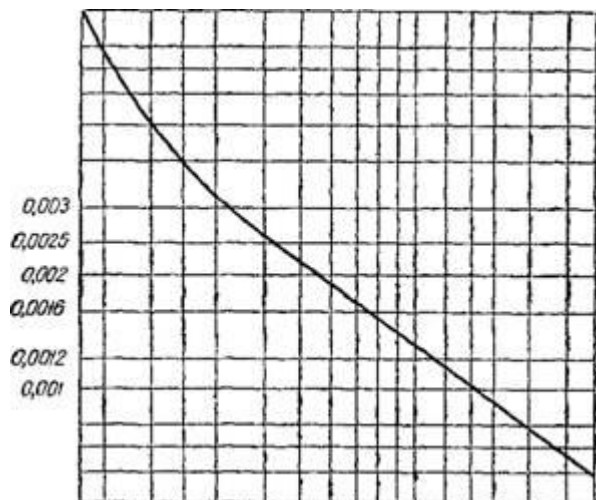
Рисунок 5. Минимальные уклоны
